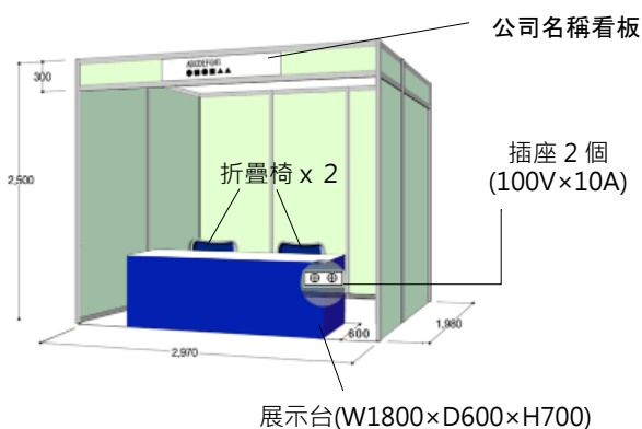
(圖2)附基本配備的標準展位 (示意圖)
